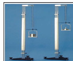
قانون هوک
