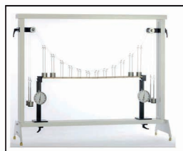
آزمایش پل معلق
