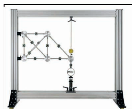
آزمایش خرپا
