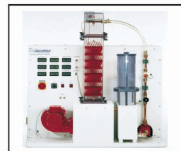
برج خنک کن تر
