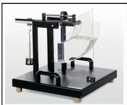
آزمایش مرکز فشار
